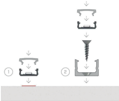
Instrucciones de instalación del perfil D con una cobertura High; (1) cinta de doble cara (2) un pasador de ensamblado y tornillo MINI
