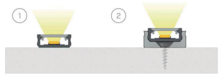
Resultado final del montaje del perfil D con cobertura básica: (1) cinta de doble cara (2) un pasador de ensamblado y tornillo MINI
