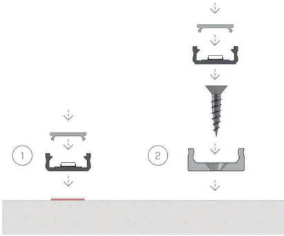
Instrucciones de instalación del perfil D con cobertura básica: (1) cinta de doble cara (2) un pasador de ensamblado y tornillo MINI
