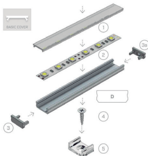
Esquema de montaje del Perfil D Basic (1) una cobertura básica, (2) una tira de LED, (3) una tapa de extremo con agujero, (3a) una tapa de extremo sin agujero, (4) un tornillo de montaje, (5) una placa de montaje MINI para el perfil
