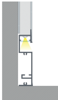
El resultado final de montaje de perfil de base FLARO con difusor BASIC y pieza de perfil enyesada.
