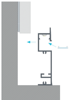
Manual de instalación para perfil base FLARO con difusor BASIC.
