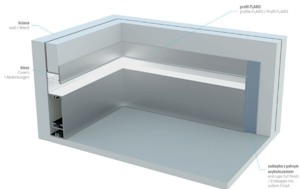
Ejemplo del montaje de perfil base FLARO bajo un ángulo y en el punto de conexión entre paredes.
