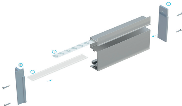
El esquema de montaje de elementos de sistema de iluminación usando perfil FLARO (1) difusor BASIC, (2) tira LED, (3) tapón con acabado recto, (3) tapón con acabado completo.
