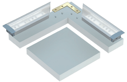
Conexión de perfiles INSILEDAs usando conector angular en ranura abierta.
