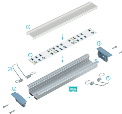
Esquema de montaje de elementos del sistema de iluminación usando perfil INSILEDAs y (1) difusor DOUBLE (2) tiras LED, (3) tapones con agujero y (4) resorte de montaje.
