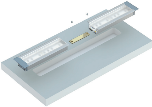
Conectando perfiles INSILEDAs usando conector recto con ranura abierta.
