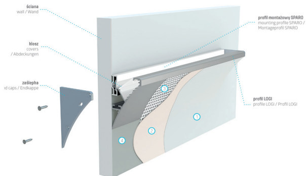
Etapas de montaje de perfil LOGI en la pared [1 pintura, 2 yeso, 3 red, 4 cartón yeso].
