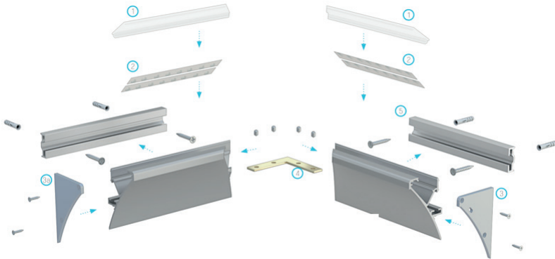
El esquema de montaje de elementos del sistema de iluminación usando perfil LOGI, (1) difusor DOUBLE, (2) tira LED, (3) tapón LOGI con agujero, (3a) tapón LOGI sin agujero, (4) conector angular, (5) perfil de montaje SPARO.
