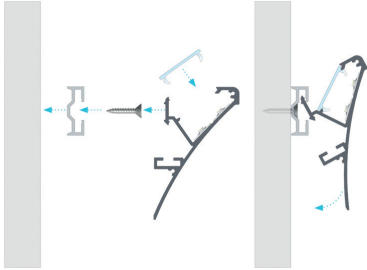
Principio de montaje de perfil LOGI con difusor DOUBLE usando perfil de montaje SPARO.
