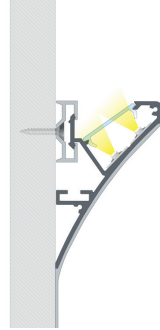
El resultado final de montaje de perfil LOGI con difusor DOUBLE usando el perfil de montaje SPARO con pieza enyesada de perfil.
