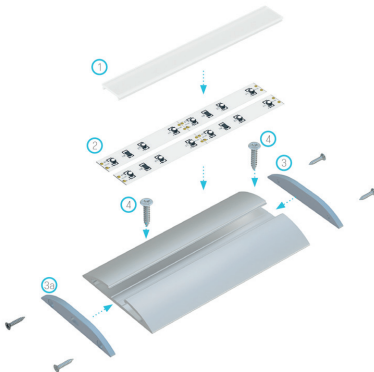
Esquema de montaje para elementos de sistema de iluminación usando (1) difusor BASIC, (2) dos tiras LED, (3) tapón sin agujero, (3a) tapón con agujero, (4) tornillos de montaje.
