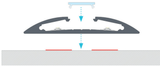
Instrucciones de instalación de perfil RETO con difusor BASIC usando la tira LED de doble cara.
