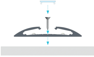
Instrucciones de instalación para el perfil RETO con difusor BASIC usando el tornillo de montaje.
