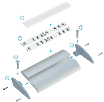
Esquema de montaje para elementos de sistema de iluminación usando (1) difusor BASIC, (2) dos tiras LED, (3) tapón con soporte de 30 grados sin agujero, (3a) tapón con soporte de 30 grados y con agujero (4) tornillos de montaje.
