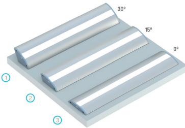
Instalación de perfil RETO usando (1) tapón de 30 grados, (2) tapones de 15 grados, (3) tapones de 0 grados.
