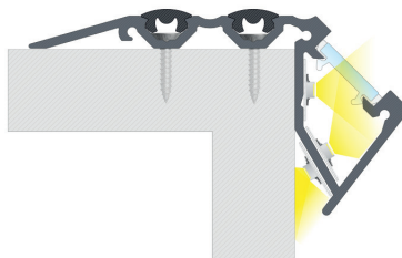
El resultado final de montaje de perfil de escalera SCALA con difusor TERRA filamento antideslizante ANTI.
