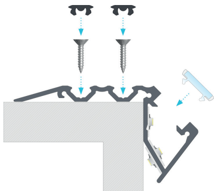
Instrucción de montaje de perfil de escalera SCALA con difusor TERRA y filamento antideslizante ANTI.
