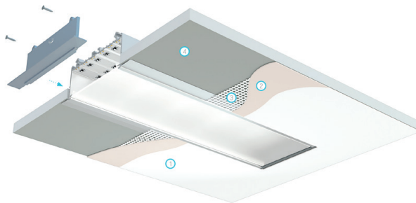
Estadios del montaje de perfil SORGA en desarrollo directo [1 pintura, 2 yeso, 3 red, 4 cartón yeso].
