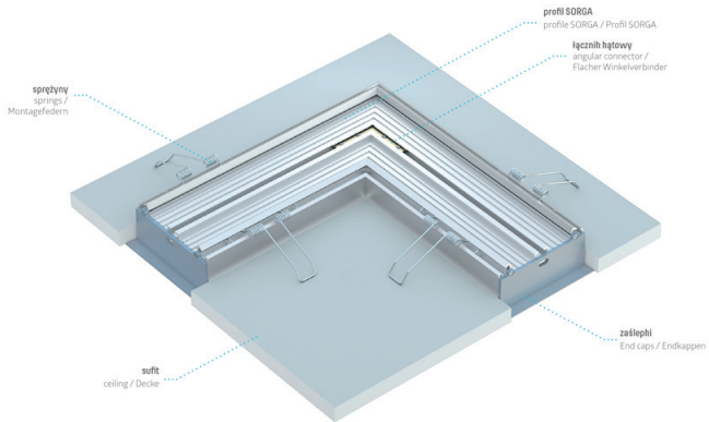
El resultado final de montaje de perfil SORGA con difusor SUPER WIDE usando muelles de montaje y conector angular. Vista isométrica desde arriba.
