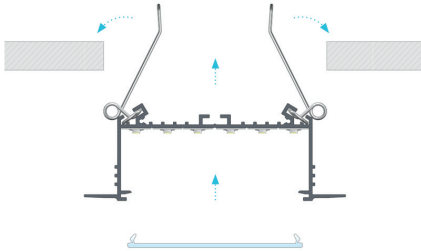
Manual de instalación de perfil SORGA con difusor SUPER WIDE, usando muelles de montaje.
